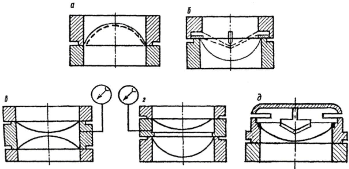
Рис. 1. Типовые мембранные предохранительные устройства:
