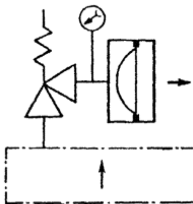
Рис. 4. Схема установки МПУ за клапаном
