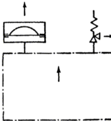
Рис. 3. Схема установки МПУ параллельно с клапаном
