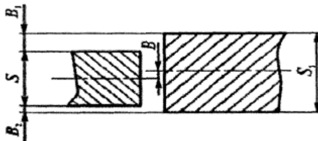
Рисунок 15. Смещение кромок
