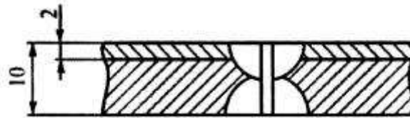
Рисунок 18. Образец для испытания на ударный изгиб сварных соединений из двухслойных сталей.
