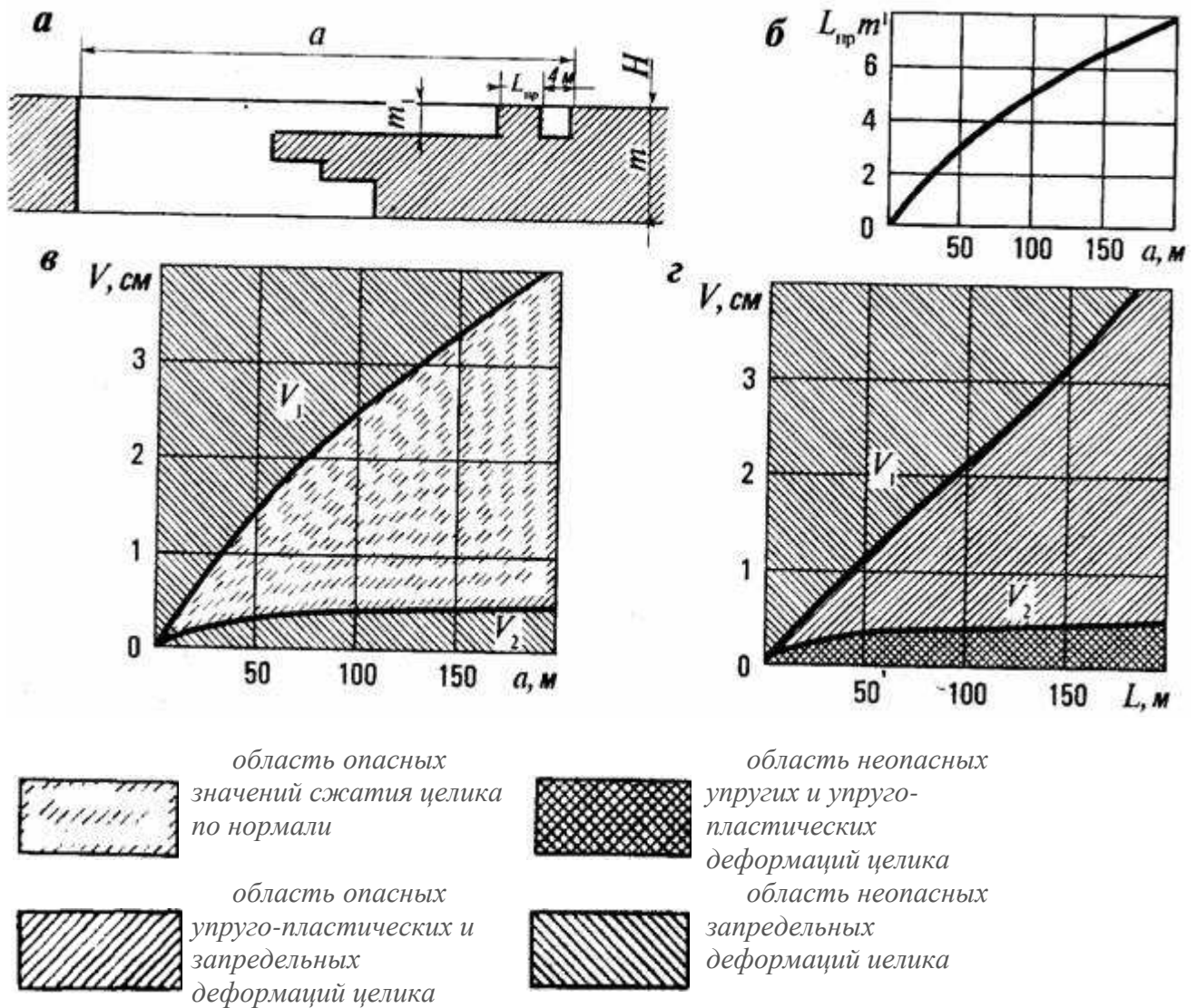
Рис. 15. Оценка состояния податливых целиков: а — расчетная схема, б — зависимость предельного размера целика от ширины выработанного пространства, в — зависимость величины сжатия целика по нормали от ширины выработанного пространства, г — номограмма для оценки состояния целика по величине сжатия по нормали; m' — вынимаемая мощность слоя; H — глубина разработки
