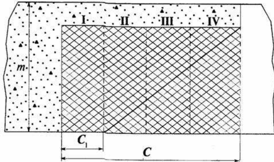
Рис. 14. Построение защищенной зоны при опережающей отработке рудного тела. I—IV — номер блока, панели, полосы, ленты
