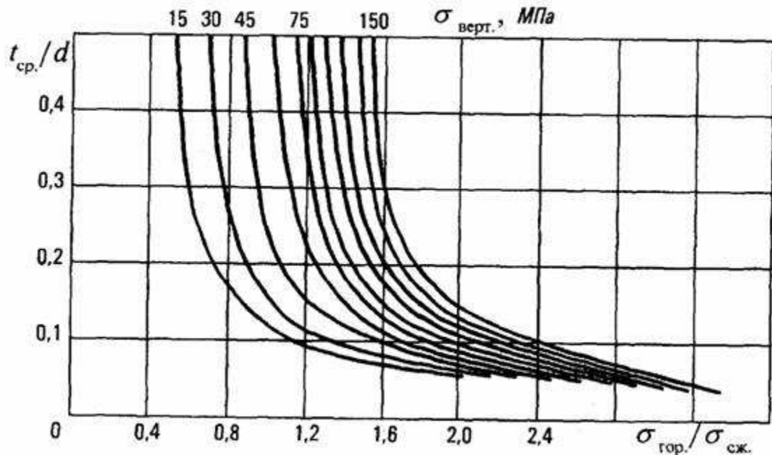
Рис. 12. Номограмма для оценки напряженного состояния пород \sigma_{\text{гор.}} / \sigma_{\text{сж.}} по дискованию керна по данным бурения геологоразведочных скважин при различных вертикальных напряжениях, определяемых величиной \gamma H :
