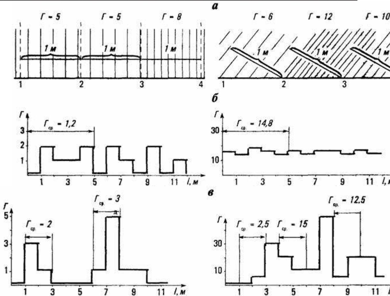
Рис. 10. Определение интенсивности трещин: а — определение плотности (числа) трещин; б, в — примеры оценки средней плотности (числа) \Gamma_{\text{ср}} трещин поперечной направленности по длине участка выработки l
