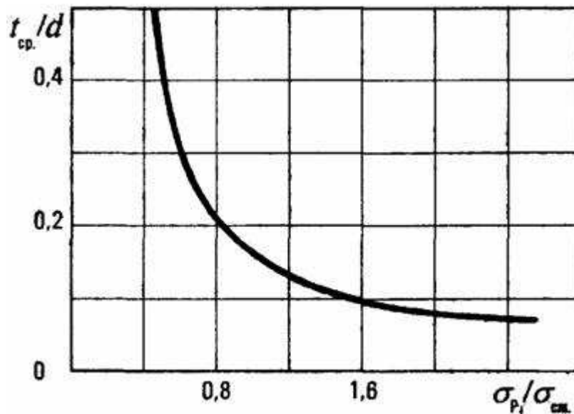
Рис. 7. Номограмма для определения напряжений в максимуме зоны опорного давления по дискованию керна
