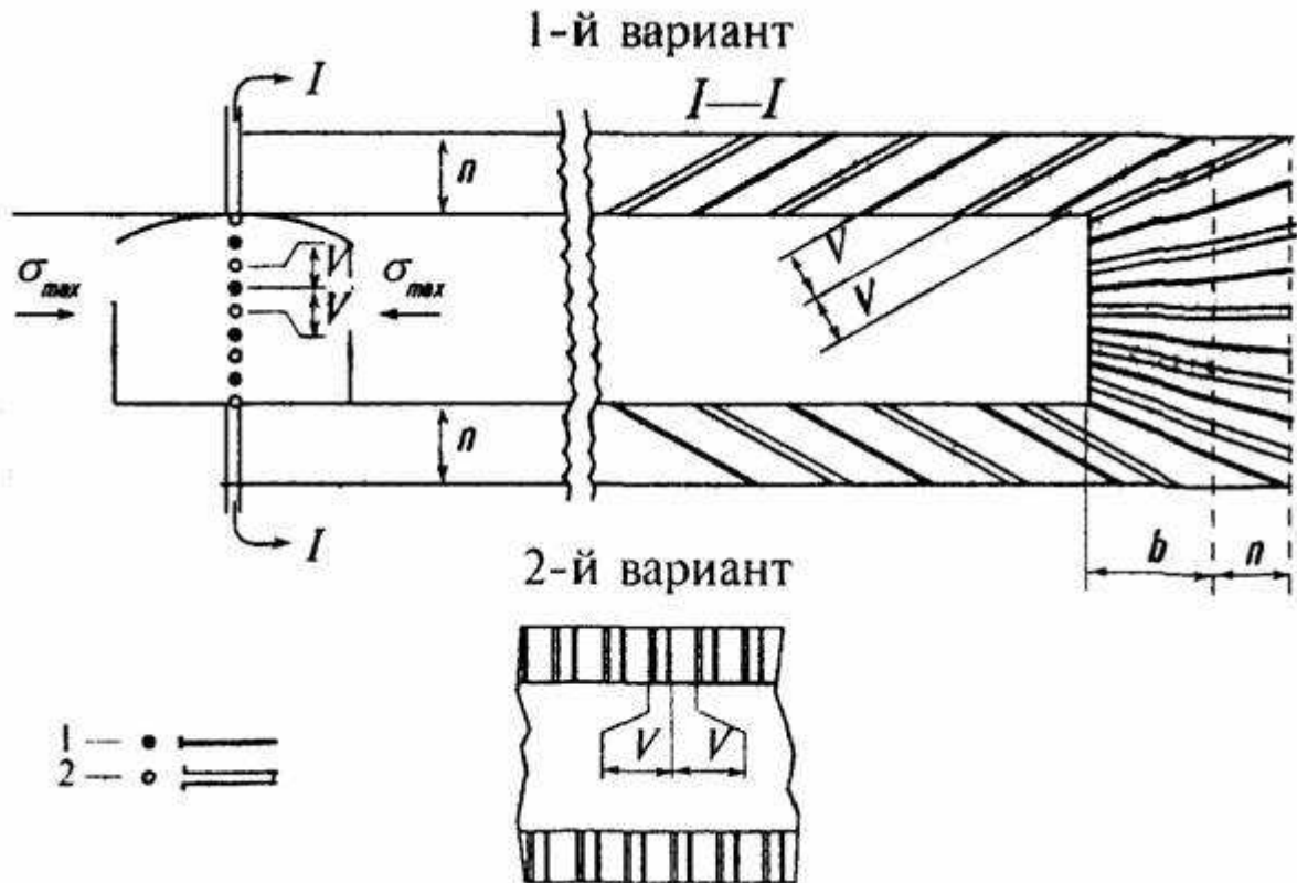
Рис. 3. Схемы применения камуфлетных и компенсационных скважин (шпуров). 1 — камуфлетный шпур; 2 — компенсационная скважина
