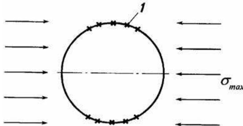
Рис. 16. Ориентировка участков разрушения пород 1 в сечении выработки относительно наибольших сжимающих напряжений
