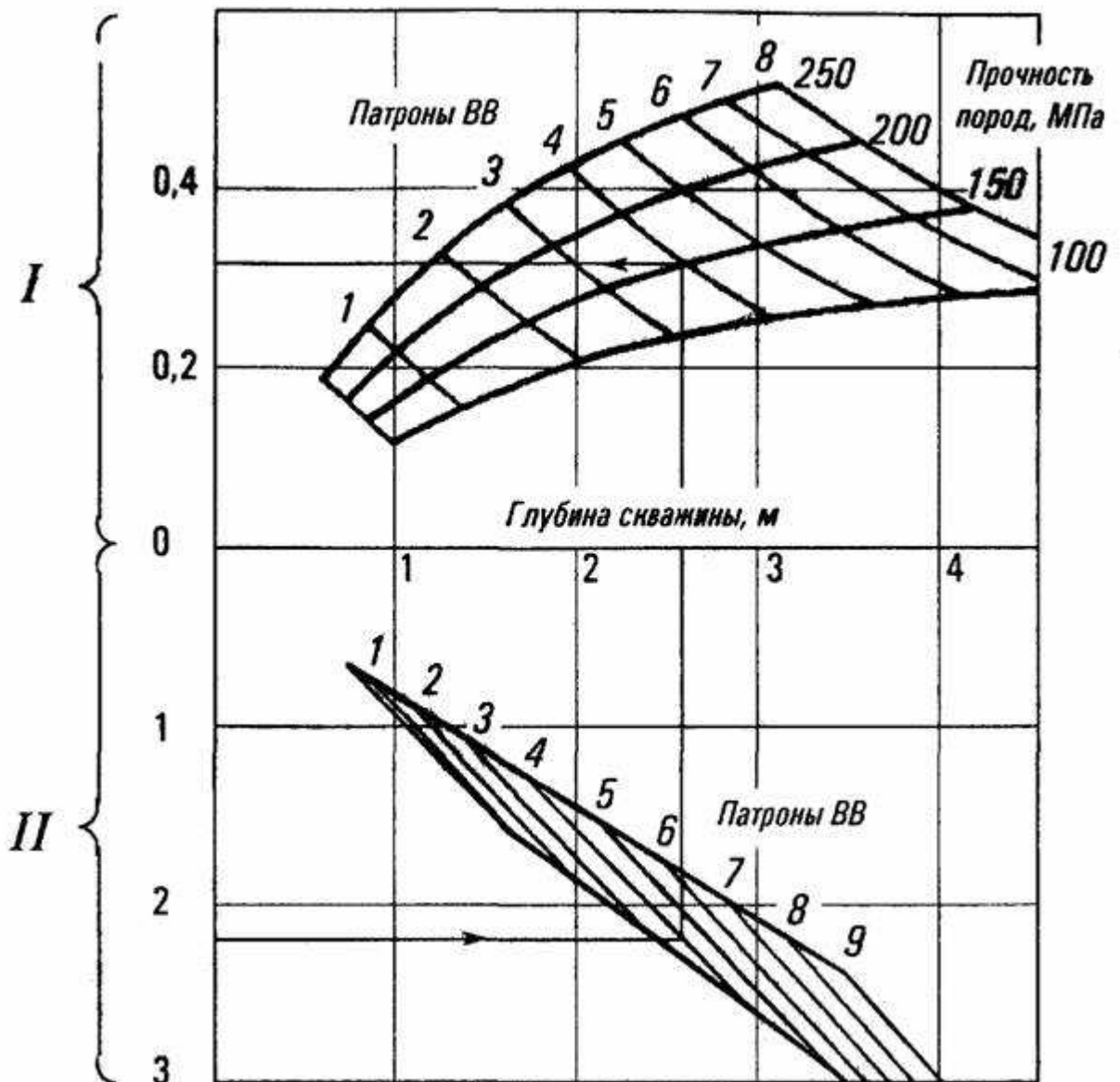
Рис. 2. Номограмма для определения параметров камуфлетного взрывания ряда шпуров (масса патронов ВВ 0,2 кг) I — относительная длина заряжаемой части скважины; II — расстояние до максимума напряжений, м.
