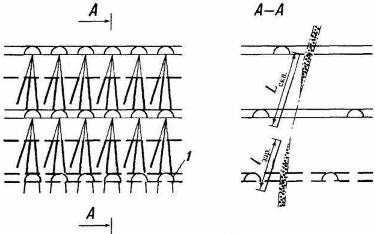
Рис. 4. Схема расположения скважин вблизи тектонического нарушения. 1 — проектируемый горизонт; L_{скв.} — длина скважины; l_{зар.} — длина заряда: l_{зар.} \leq 0,75 L_{скв.}
