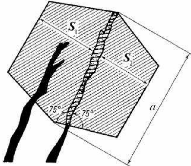
Рис. 13. Построение защищенной зоны
