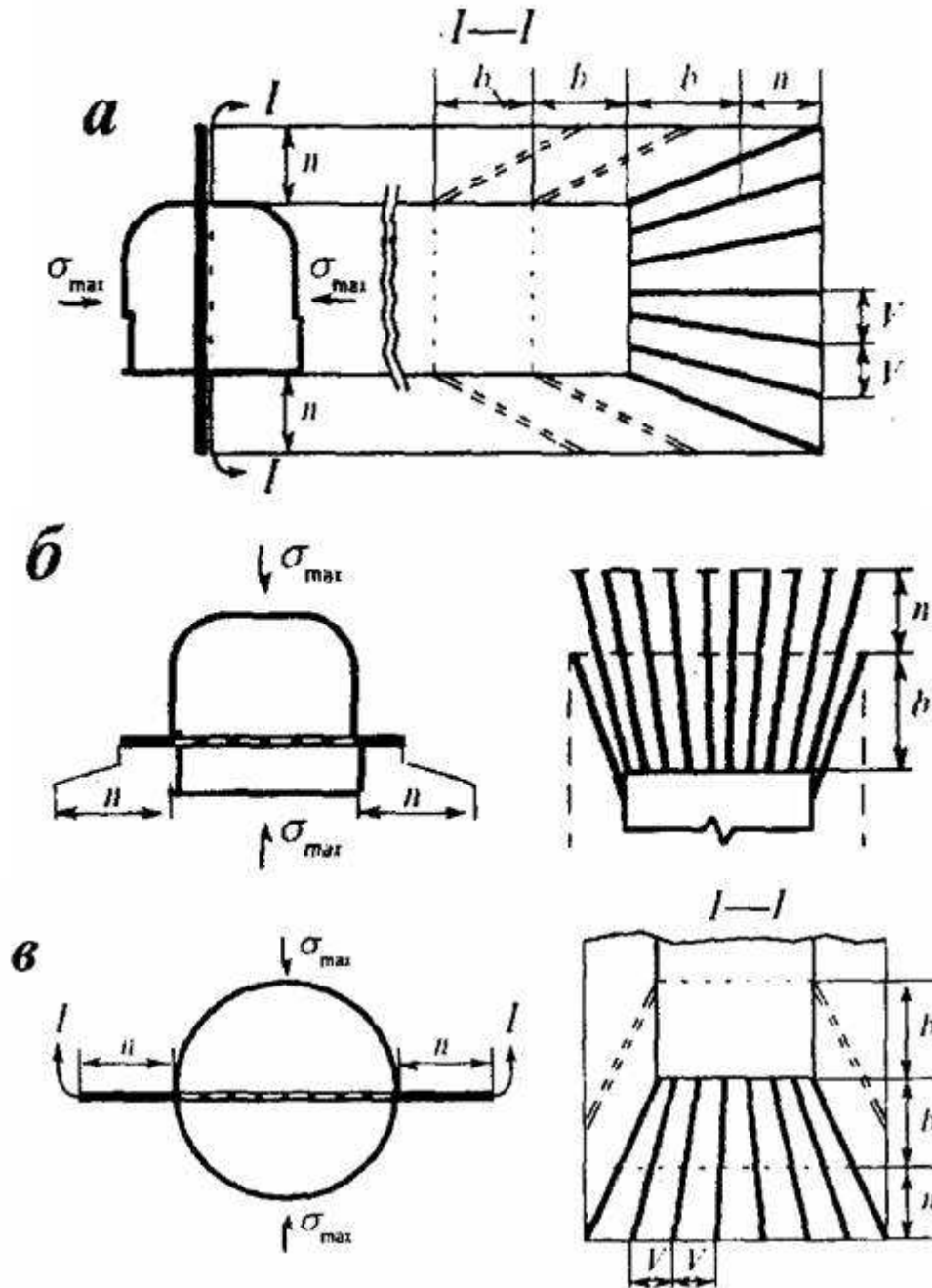
Рис. 1. Схемы камуфлетного взрывания по рядам шпуров:
