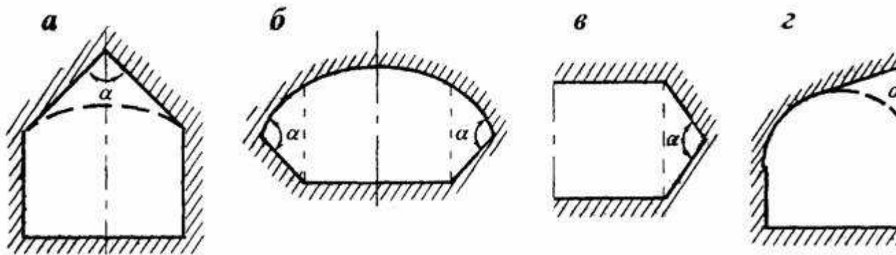
Рис. 5. Полигональная форма выработок при расположении мест разрушения: а — в кровле, б — в стенках, в — в забое, з — в сопряжении кровли со стенкой; а \angle 100^\circ — угол разрушения
