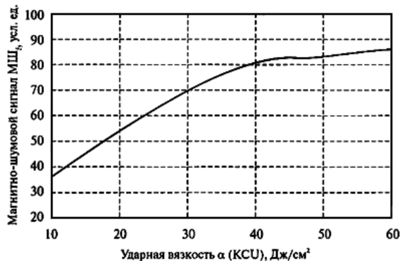
Рис.И.3. Зависимость ударной вязкости (КСУ) от магнитно-шумового сигнала. Прибор "ПИОН-01" зав. N 12. Ст 3, 4
