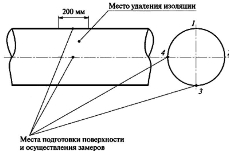
Рис.И.4. Схема расположения мест замера
