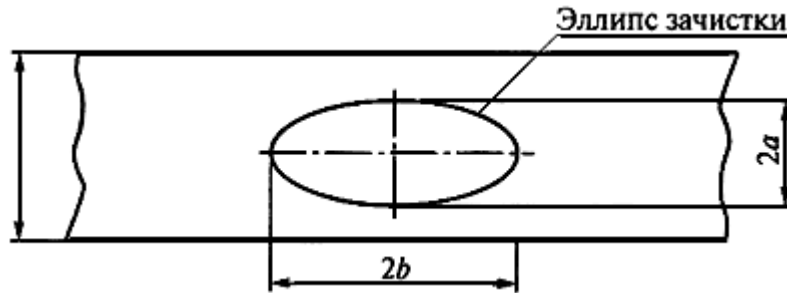
Рис.3.2. Схема зачистки на трубопроводе
