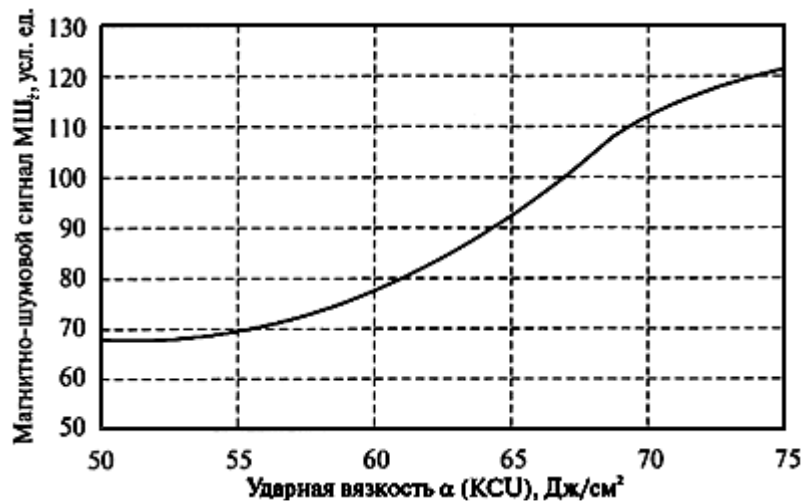
Рис.И.2. Зависимость ударной вязкости (КСУ) от магнитно-шумового сигнала. Прибор "ПИОН-01" зав. N 12. Сталь 10
