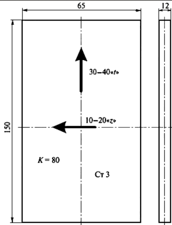
Рис.И.5. Эскиз эталонного образца для настройки прибора "ПИОН-01"
