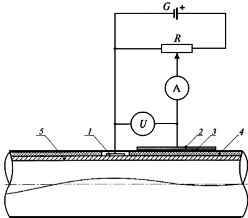
Рис.Ж.1. Электрическая схема измерения переходного сопротивления изоляционного покрытия
