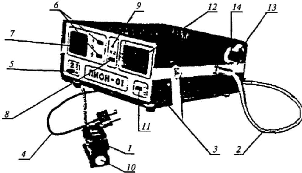
Рис.И.1. Магнитно-шумовой прибор "ПИОН-01":
