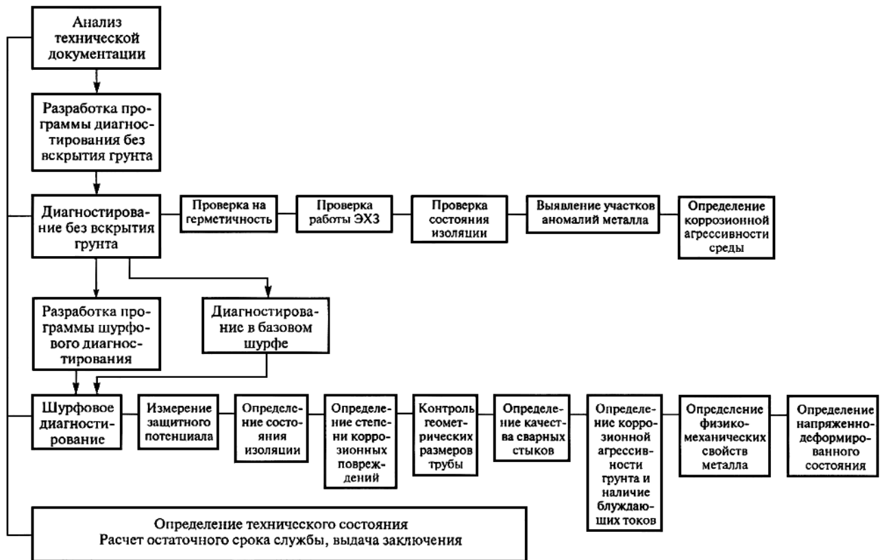
Рис.1. Схема планового диагностирования подземных газопроводов
