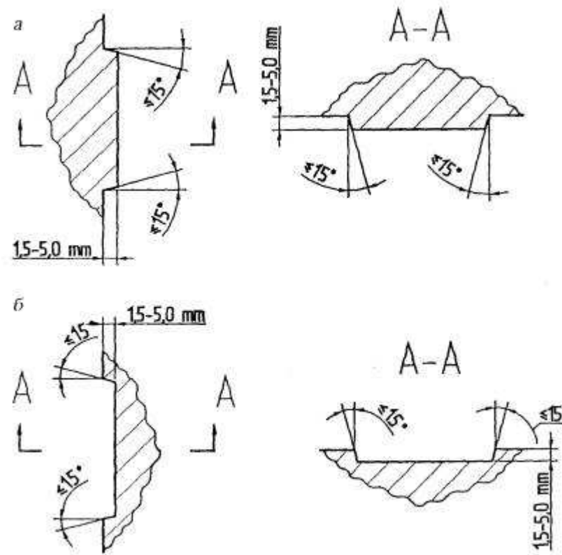
Рис. 1 . Скосы краев и впадин:
