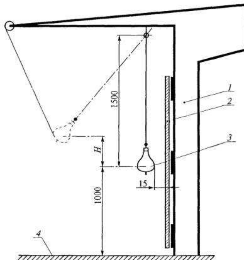
Рис. 1 . Испытательный стенд:
