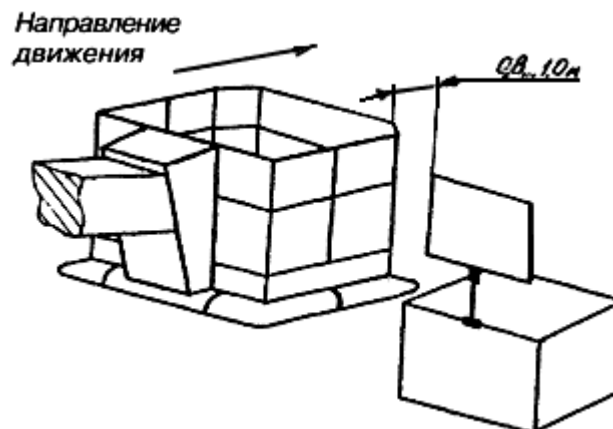
Рисунок 1. Схема положения люльки АПК относительно приспособления "щит-препятствие" при перемещении колен стрелы относительно друг друга
