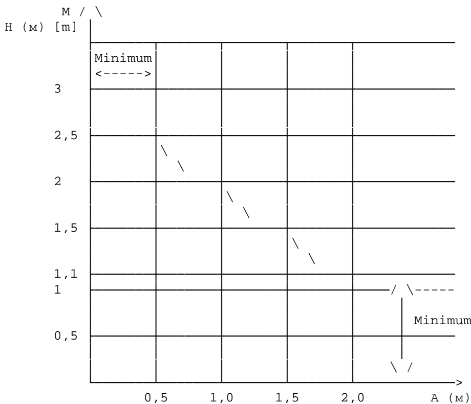
Рис. 1. Расстояние до движущихся элементов лифта (не приводится)
