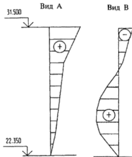
Эпюра деформаций оси колонны К-1л
